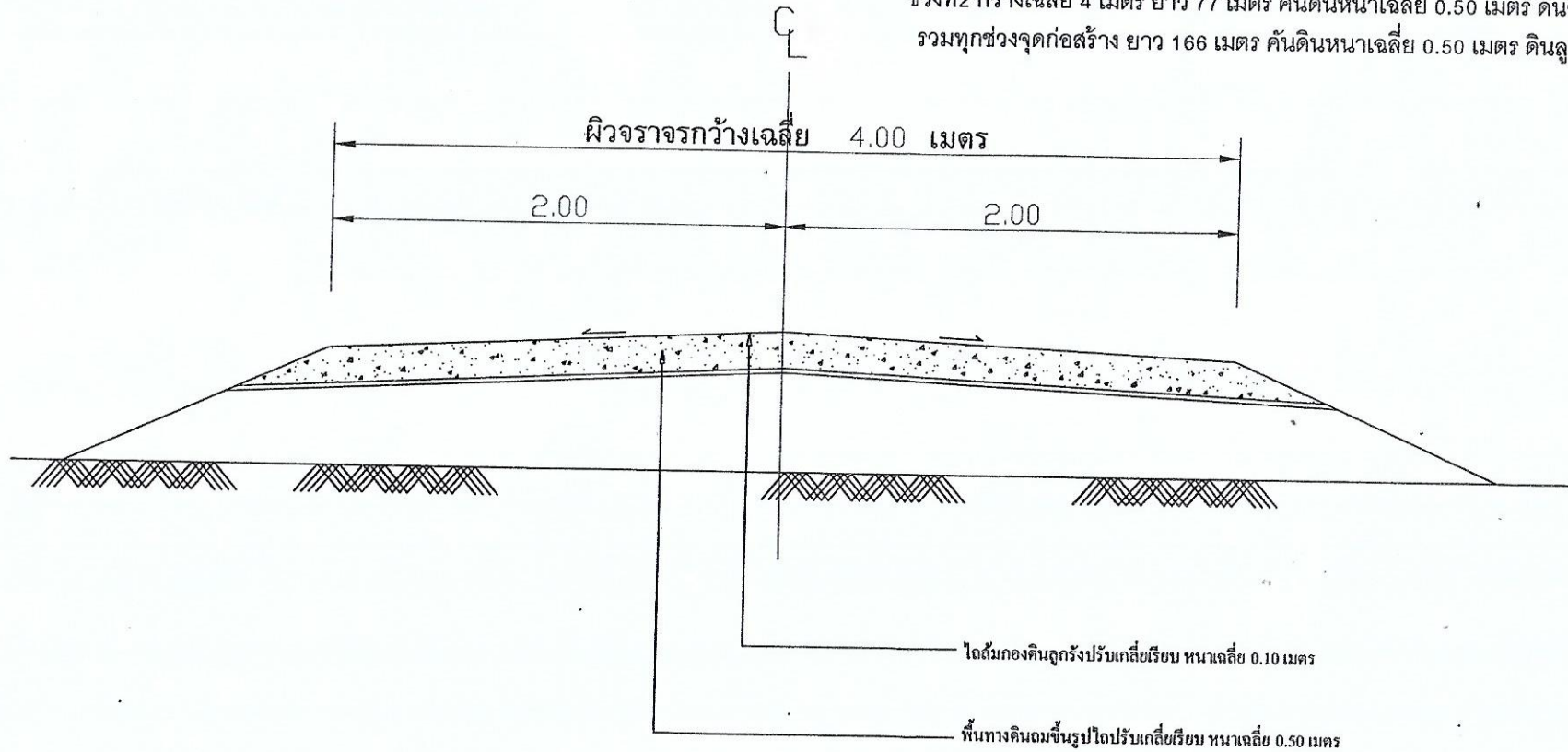
รูปตัดถนนดินลูกรัง NO TO SCALE
